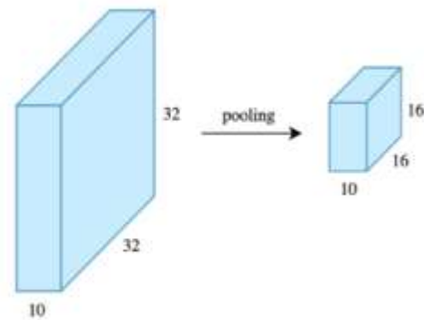
Fig. 3 Pooling layer
